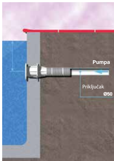
Instalacija mlaznica
