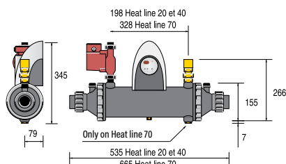
Heat Line Plus sa cirkulacionom pumpom
