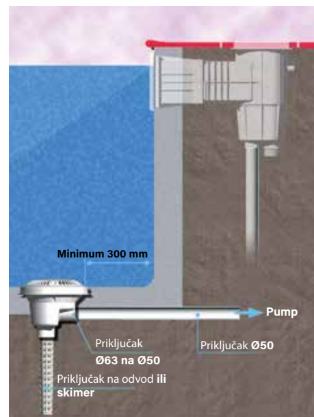
instalacija slivnika
