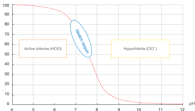
Efikasnost hlora (%)
