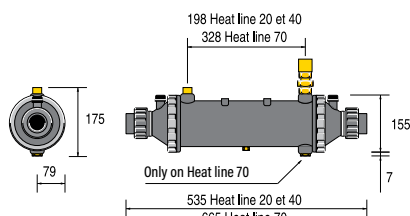
Heat Line Neopremljen
