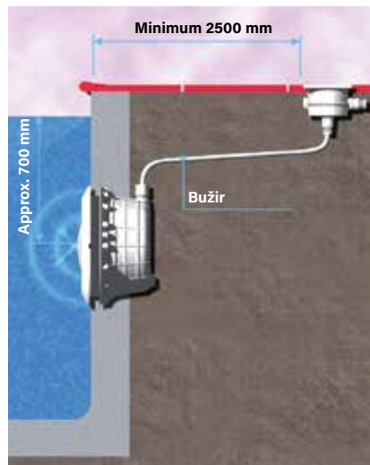
Instalacija pod vodom
