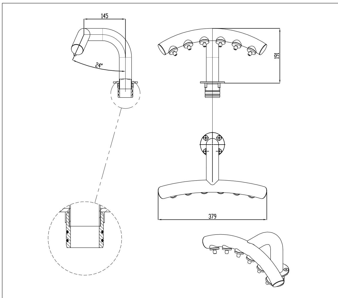
Dimenzije • Dimensiones
