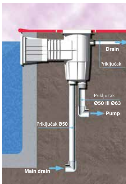
Instalacija skimera
