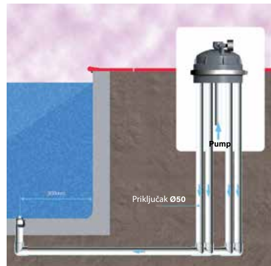
Ugradnja Net'n'Clean ventil
