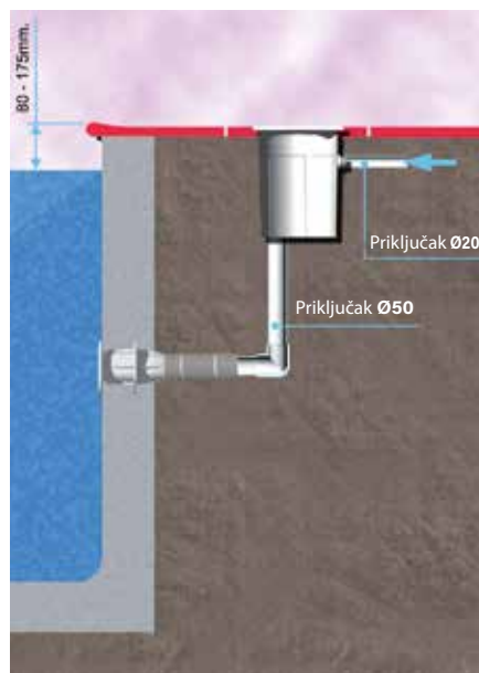
Instalacija regulatora nivoa vode
